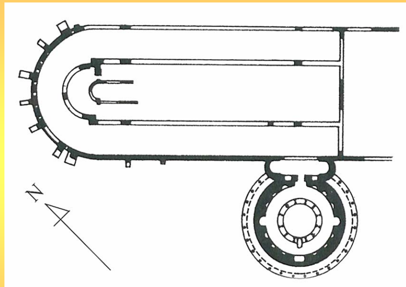
羅馬，聖依搦斯教堂（S. Agnese）與君士坦蒂娜（Constantina）墓堂，平面圖，338-353
