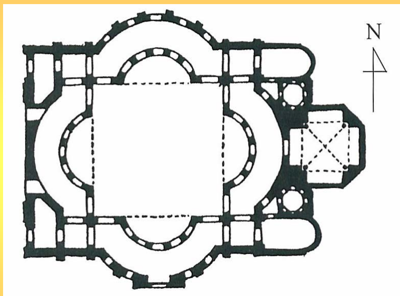
羅馬，聖勞倫佐教堂（S. Lorenzo），4世紀末，平面圖
