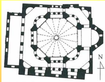
平面圖
