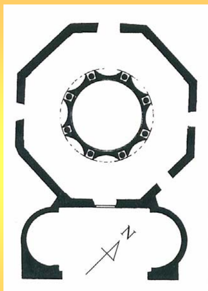
羅馬，聖若望（S. Giovanni）洗禮堂，315左右，平面圖
