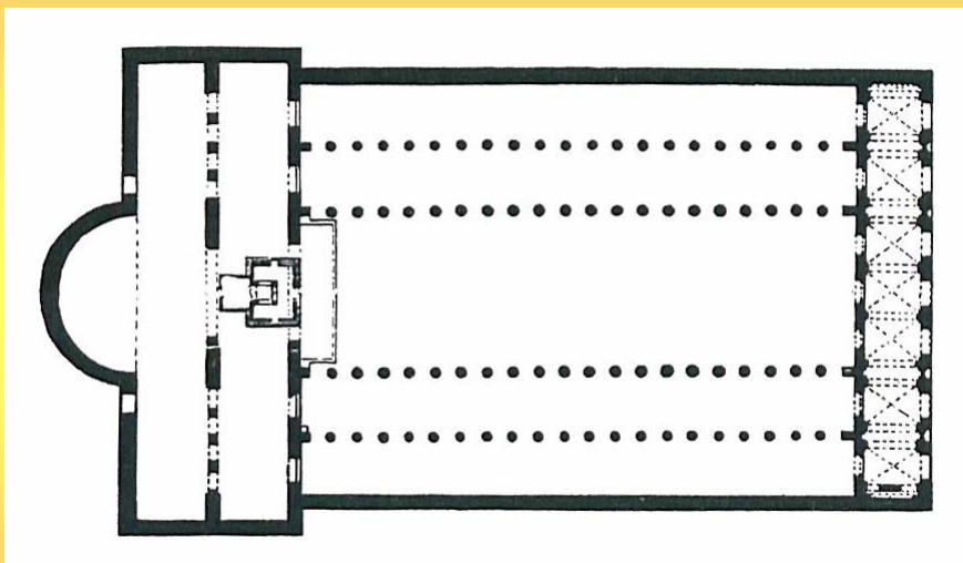
羅馬，聖保祿教堂（S. Paolo），386 始建，平面圖
