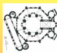
平面圖
