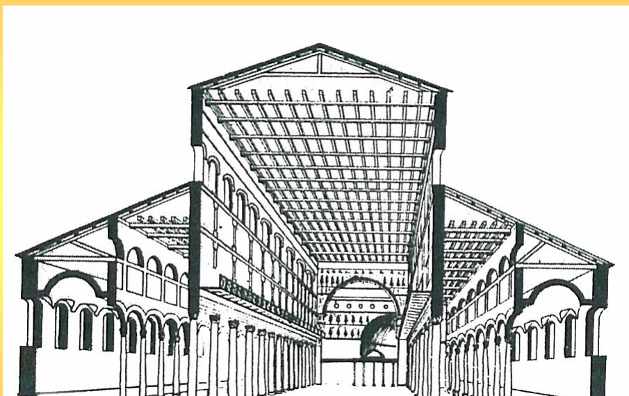
梵蒂岡，老聖彼得教堂（Old-S. Pietro），326，切面圖
