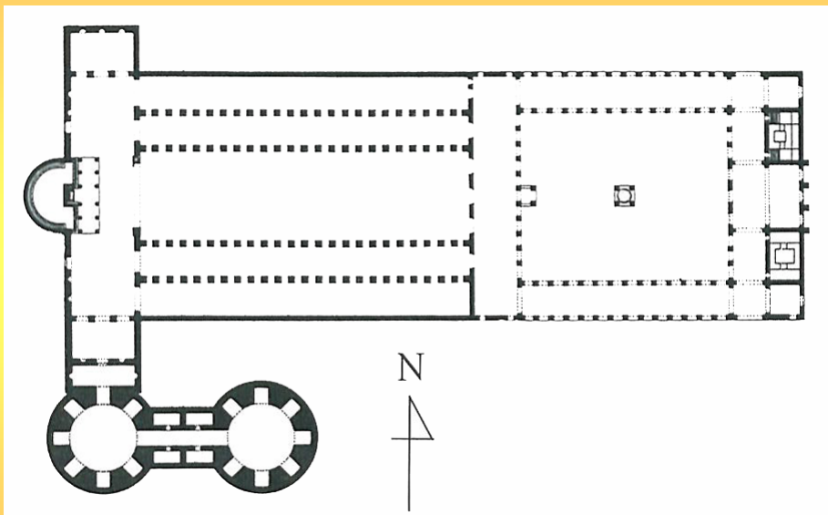
梵蒂岡，老聖彼得教堂（Old-S. Pietro），326，平面圖
