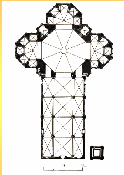
佛羅倫斯大教堂與塔（S. Maria del Fiore Duomo and Campanile），1296 始建，平面圖
