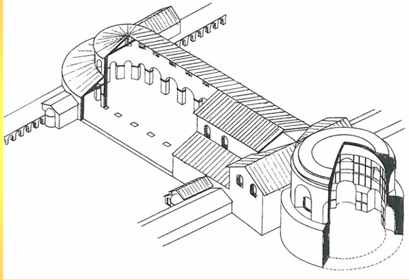
羅馬，聖馬契里諾紀念堂（SS. Marcellino e Pietro）與海倫（Helena）墓堂復元圖，4世紀上半葉
