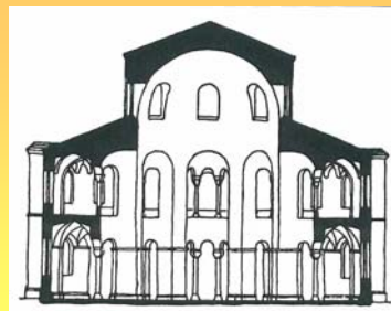
切面圖
