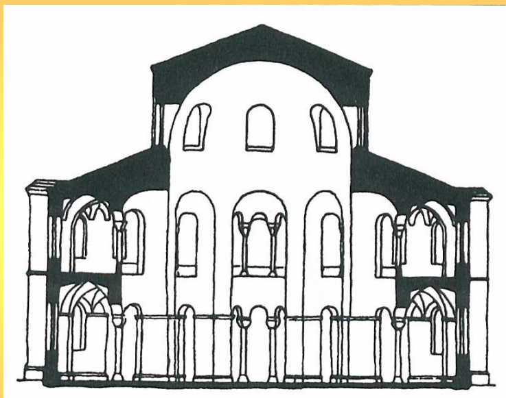
拉溫那，聖維他利教堂（S. Vitale），526-547，切面圖
