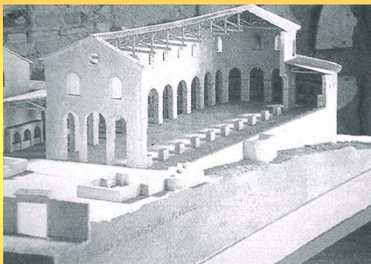
羅馬，聖西巴斯汀教堂（S. Sebastiano），剖析模型，312-340 改建
