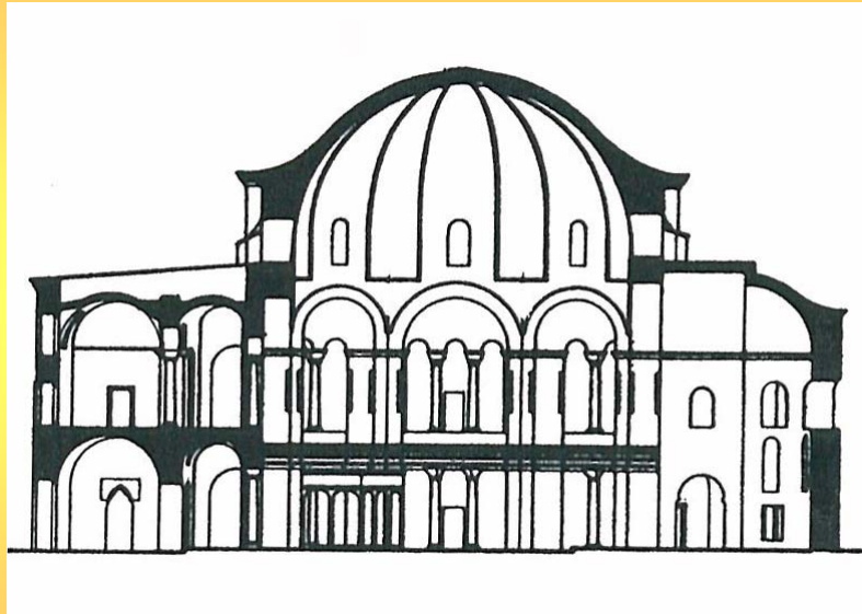
伊斯坦堡，聖西吉文與巴庫斯教堂（S. Segius and Bacchus），527 始建，切面圖
