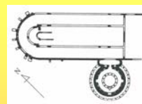
羅馬，聖依搦斯教堂（S. Agnese）與君士坦蒂娜（Constantina）墓堂，平面圖，338-353
